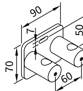
Distanzhalter 2 Einzelanlagen
