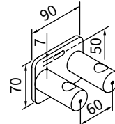
Distanzhalter 2 Einzelanlagen
