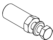
Reduzierung M 10 → M 6 / SW 13 Paket 10 Stück
