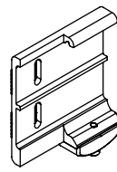
Wandhalter mit Lasche für seitliche Befestigung, links
