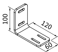
Zusatzwinkel für Nischenmontage
