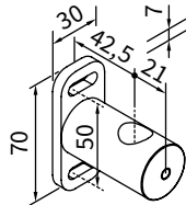
Distanzhalter
