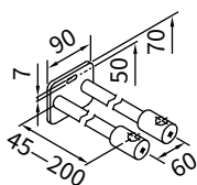
Verlängerter Distanzhalter 2 Einzelanlagen
