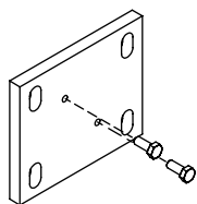
Befestigungsplatte für Wand- / Universalhalter 120 × 100 × 10 mm
