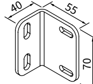
Nischenwinkel für Distanzhalter
