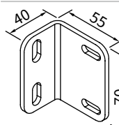
Nischenwinkel für Distanzhalter 40 × 55 × 70 mm
